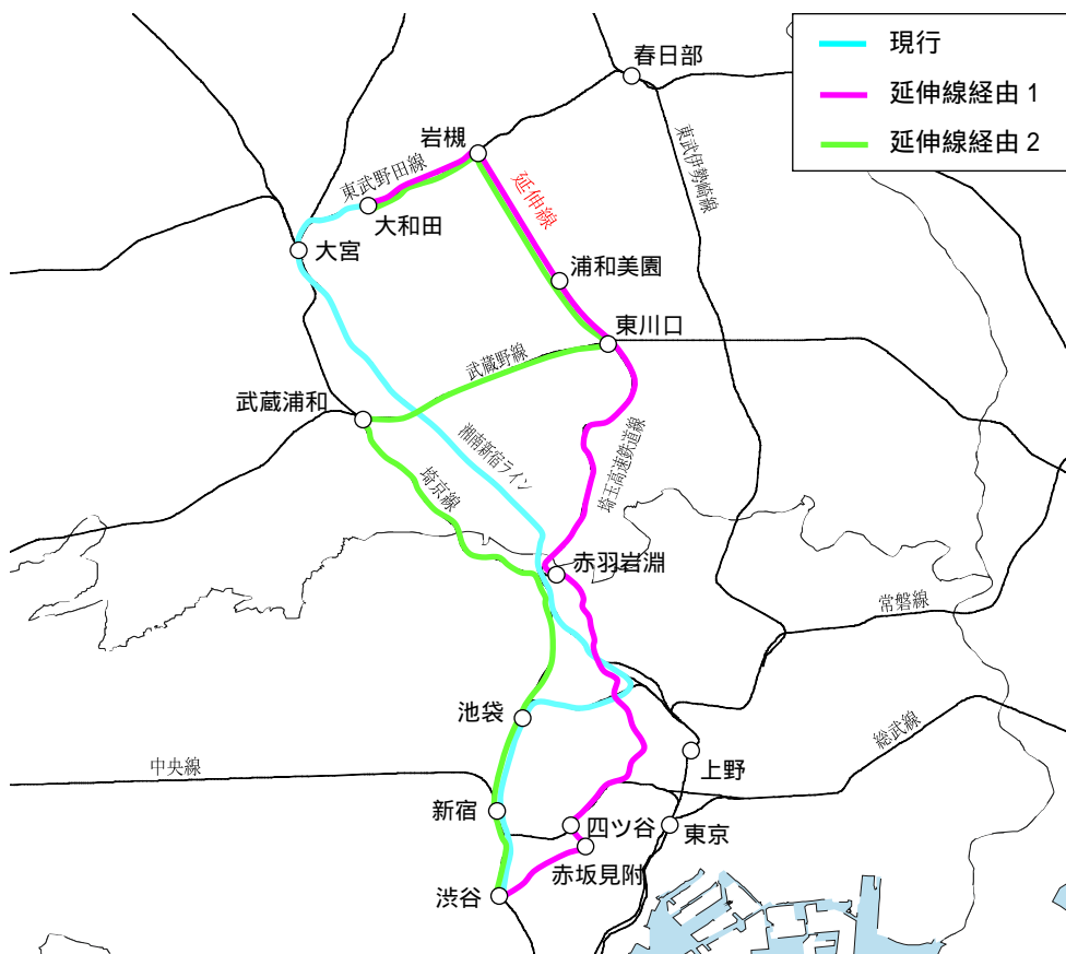
図 経路比較(大和田～渋谷)
