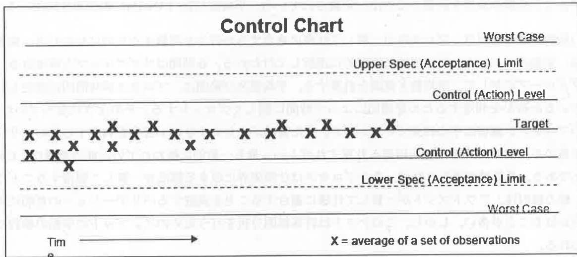
図 10 管理図
