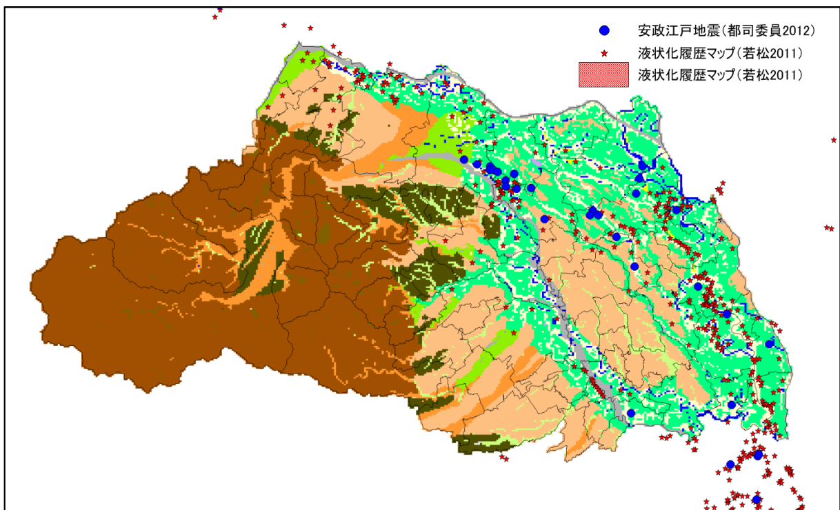
図7.1-1 歴史地震の液状化発生地点
