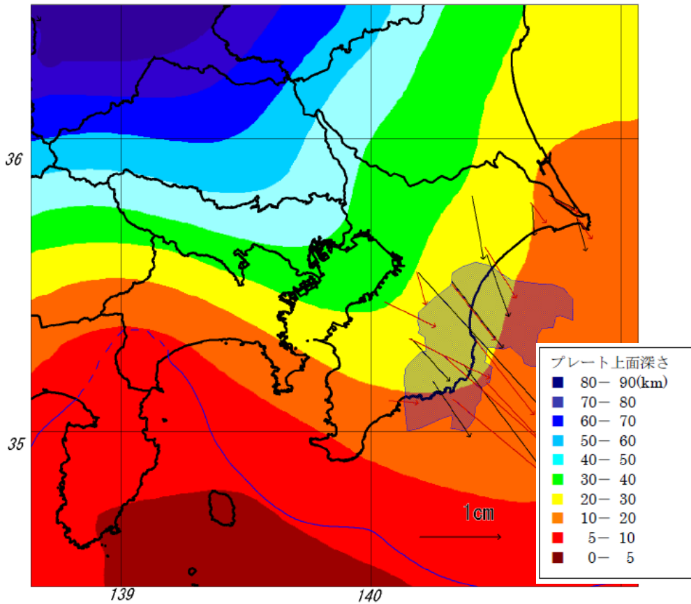
図 4.2-2 首都直下地震防災・減災プロジェクト (2012) 4 (上)・Ishida (1992) 5 (下) によるフィリピン海プレート上面深さ
