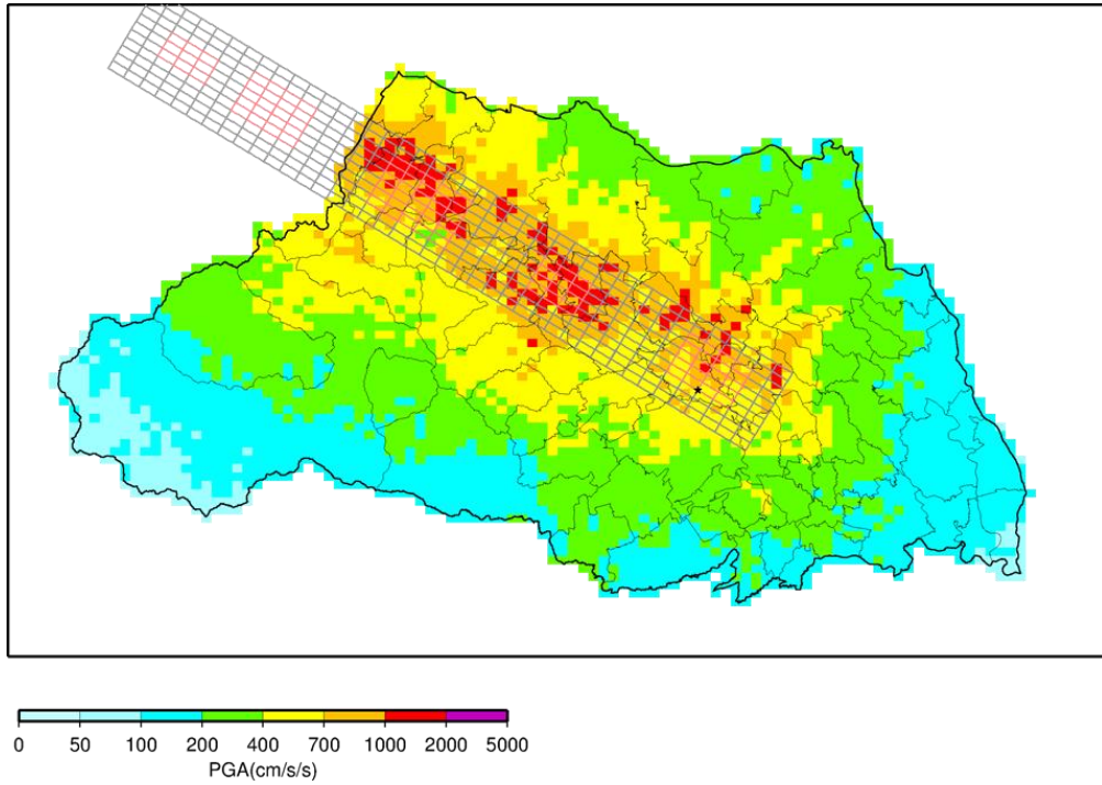
图 4.3.2-6(3) 工学的基盤加速度分布 関東平野北西縁断層帯地震(破壊開始点:南)
