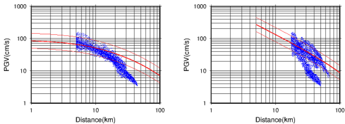
図 4.3.2-4(2) 距離減衰式（司・翠川（1999））との比較 Vs500 左：断層最短距離による最大速度 右：等価震源距離による最大速度
