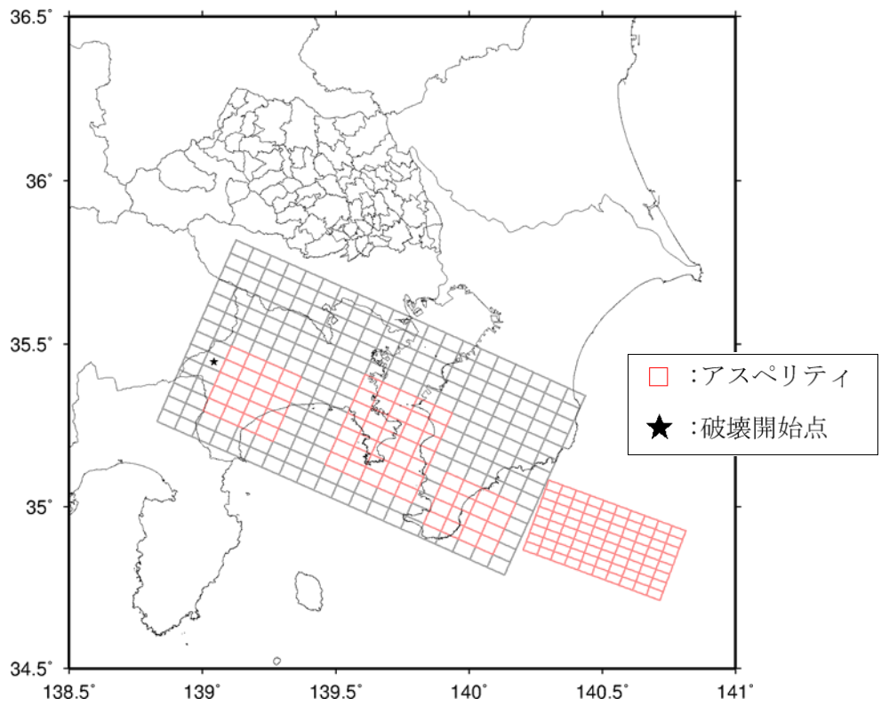
図 4.2-7 元禄型関東地震 震源断層
