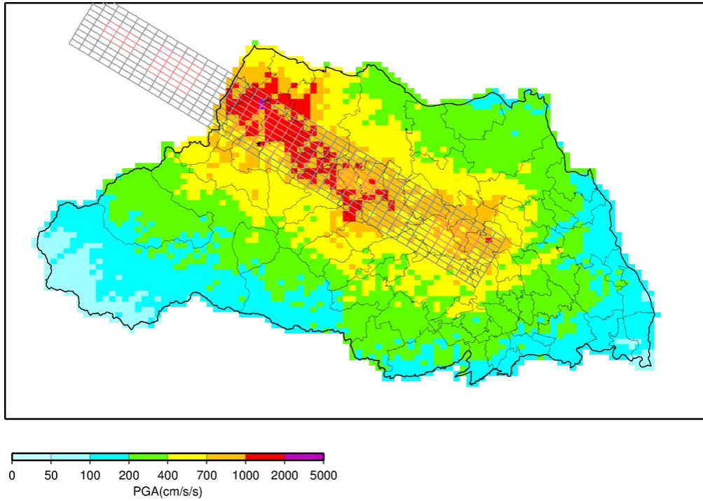
图 4.3.2-4(3) 工学的基盤加速度分布 關東平野北西緣斷層帶地震(破壞開始点:北)
