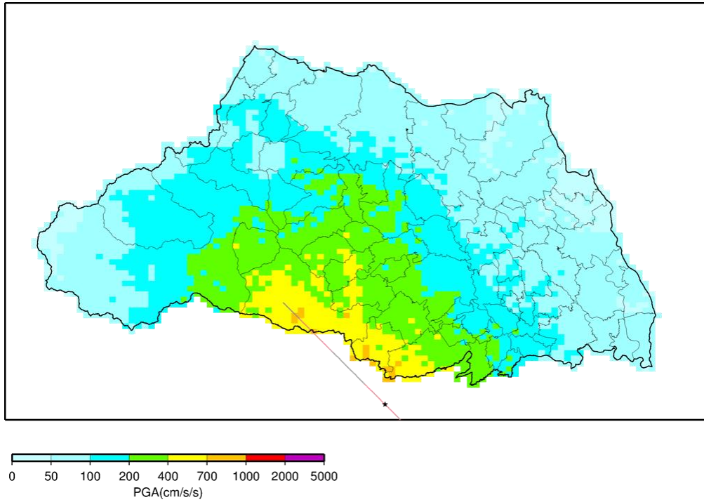
图 4.3.2-8(3) 工学的基盤加速度分布 立川断層帶地震（破壊開始点：南）
