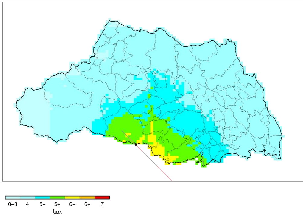
图 4.3.2-7(4) 工学的基盤震度分布 立川断層帯地震（破壊開始点：北）
