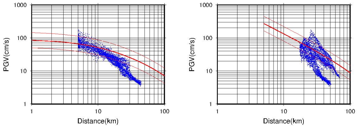
図 4.3.2-6(2) 距離減衰式（司・翠川（1999））との比較 Vs500 左：断層最短距離による最大速度 右：等価震源距離による最大速度
