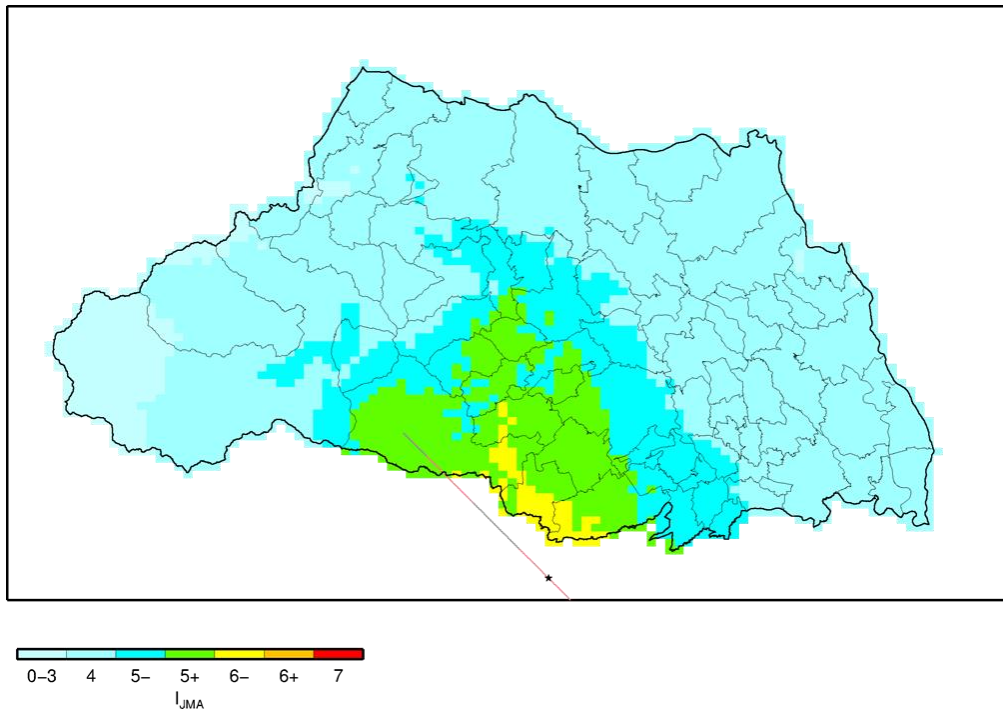
图 4.3.2-8(4) 工学的基盤震度分布 立川断層帶地震（破壊開始点：南）
