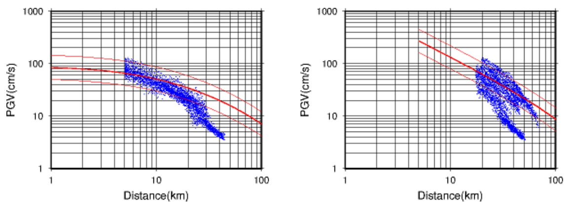
図 4. 3. 2-5 (2) 距離減衰式（司・翠川（1999））との比較 Vs500 左：断層最短距離による最大速度 右：等価震源距離による最大速度
