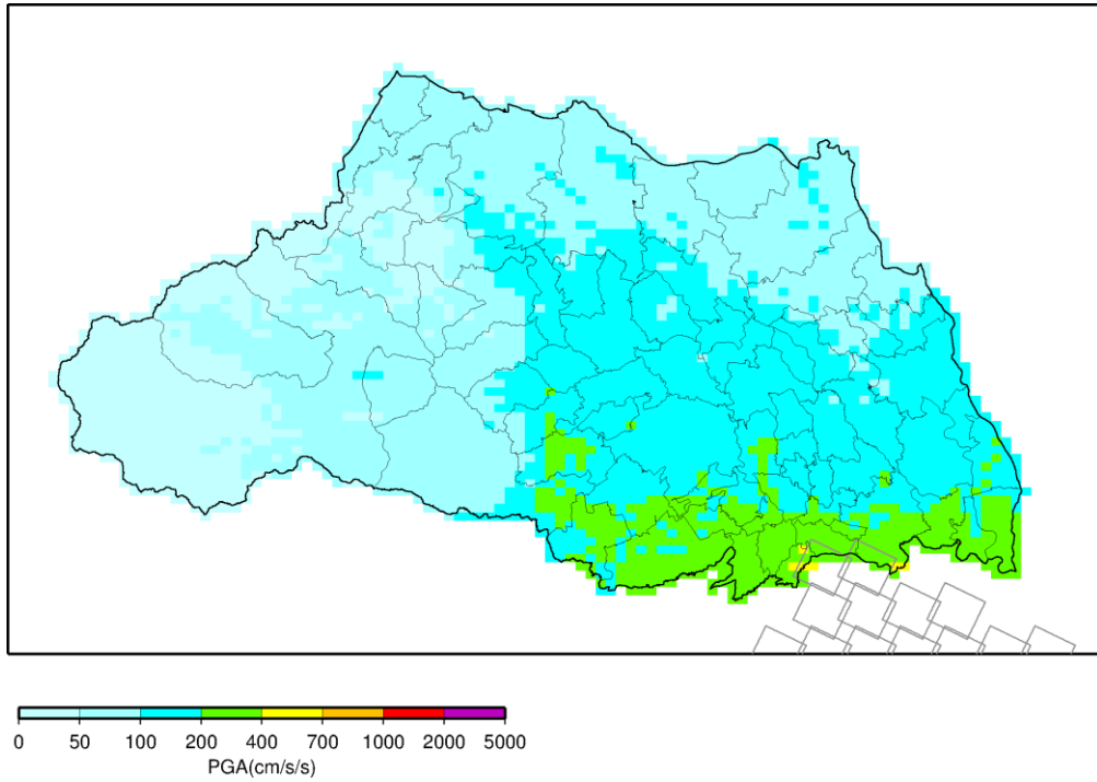
图 4.3.2-1(3) 工学的基盤加速度分布 東京湾北部地震
