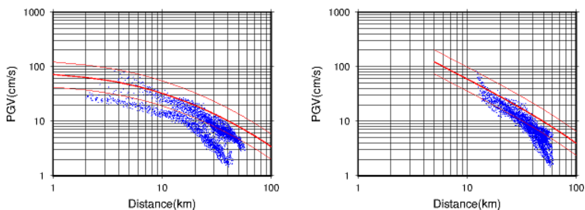
図 4. 3. 2-8(2) 距離減衰式（司・翠川（1999））との比較 Vs500 左：断層最短距離による最大速度 右：等価震源距離による最大速度
