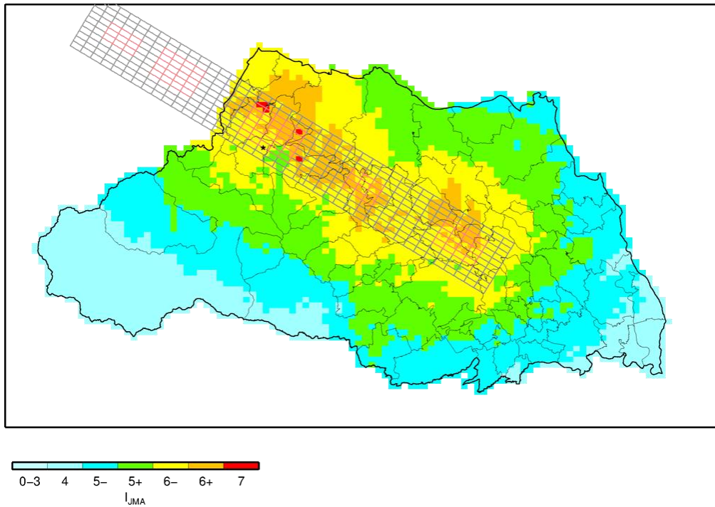
图 4.3.2-4(4) 工学的基盤震度分布 關東平野北西緣斷層帶地震 (破壞開始点:北)
