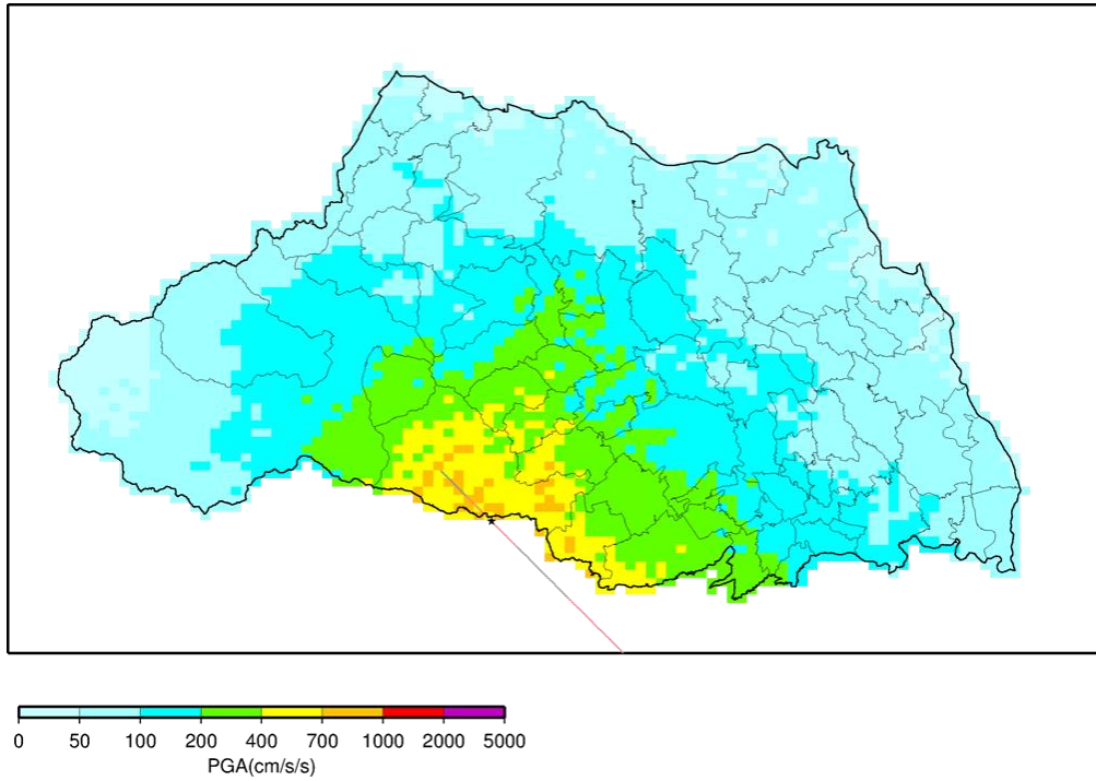
图 4.3.2-7(3) 工学的基盤加速度分布 立川断層帯地震（破壊開始点：北）
