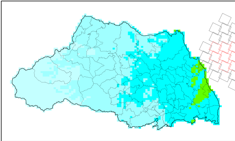
图 4.3.2-2(3) 工学的基盤加速度分布 茨城県南部地震
