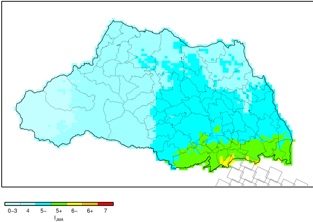
图 4.3.2-1(4) 工学的基盤震度分布 東京湾北部地震
