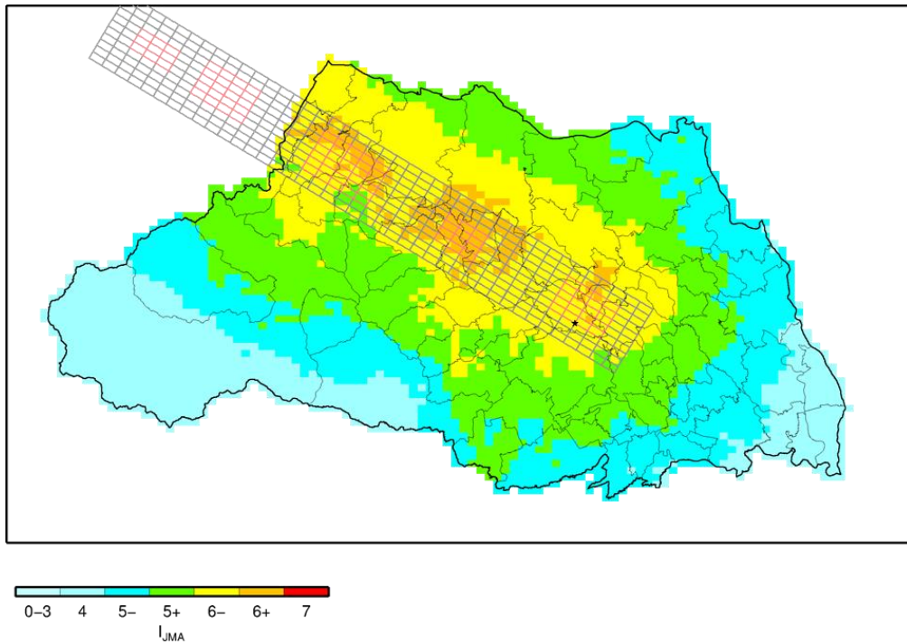
图 4.3.2-6(4) 工学的基盤震度分布 関東平野北西縁断層帯地震(破壊開始点:南)
