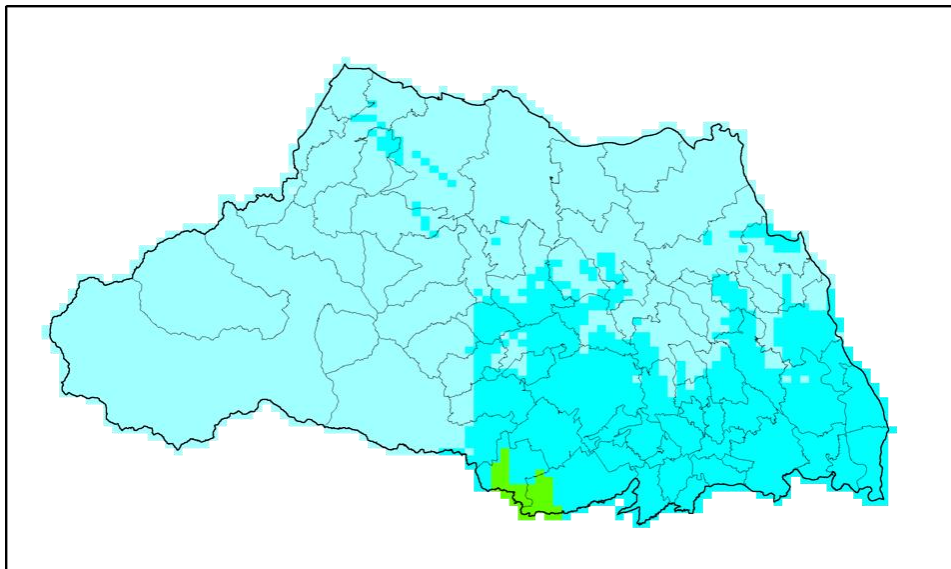
图 4.3.2-3(3) 工学的基盤加速度分布 元禄型関東地震
