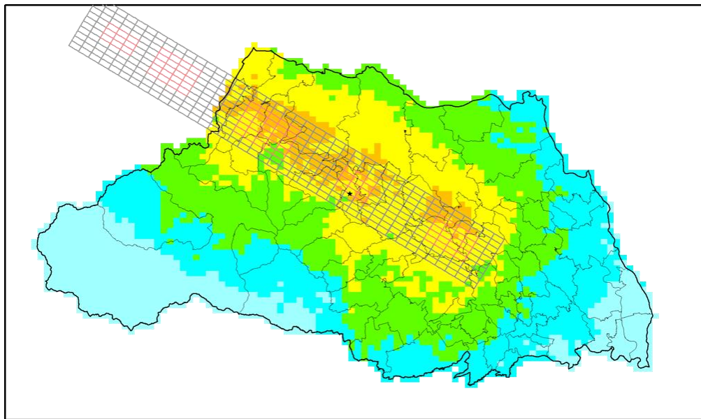
图 4. 3. 2-5 (3) 工学的基盤加速度分布 関東平野北西縁断層帯地震 (破壊開始点：中央)
