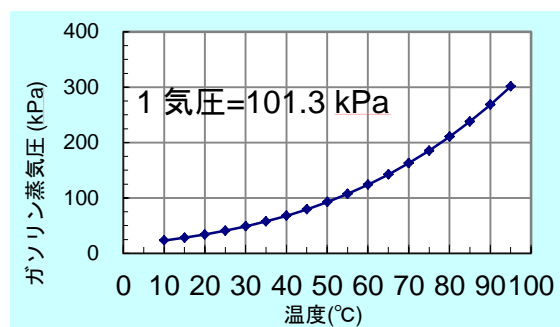
ガソリン温度と蒸気圧の関係
