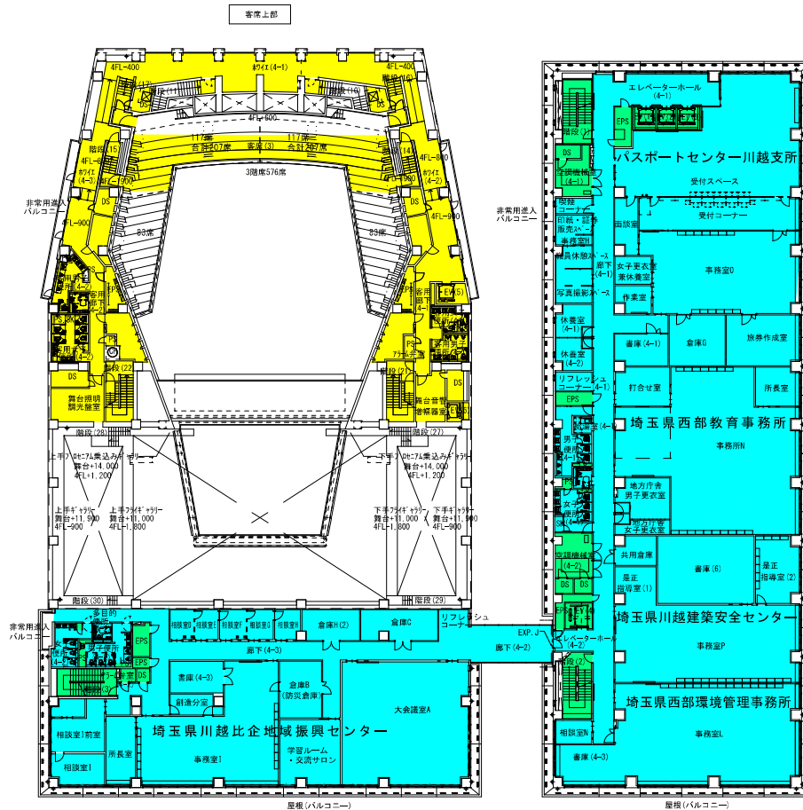
4階平面図 Scale:1/500
