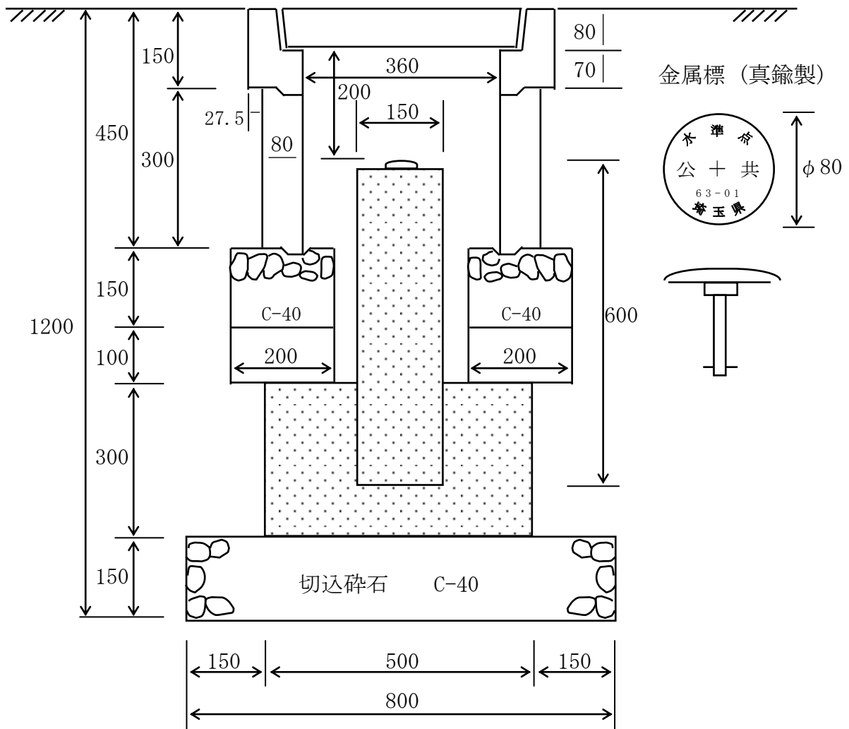
断面図
