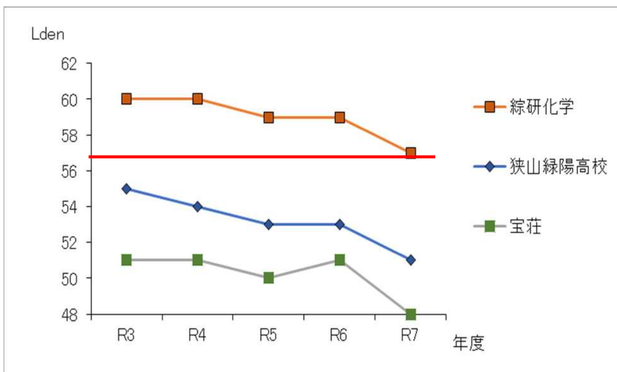
図-4 Ldenの推移（入間飛行場北側）
