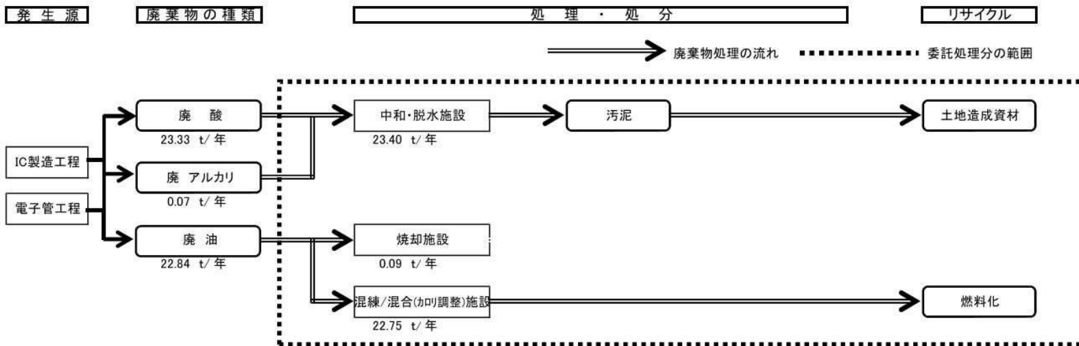
別紙2 廃棄物処理フロー図(2/2)
