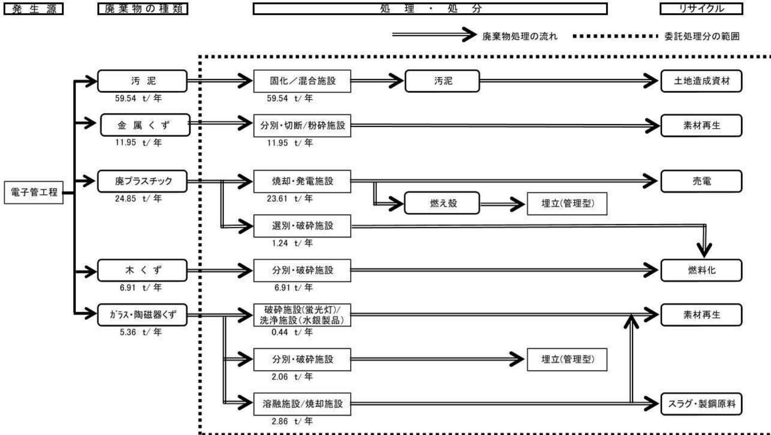
別紙2 廃棄物処理フロー図(1/2)
