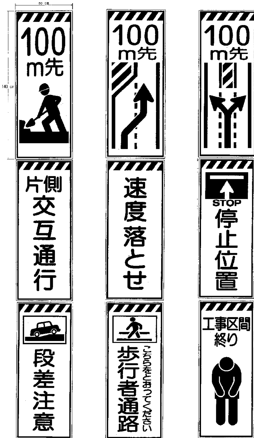
(様式-2) 工事予告標示板等
