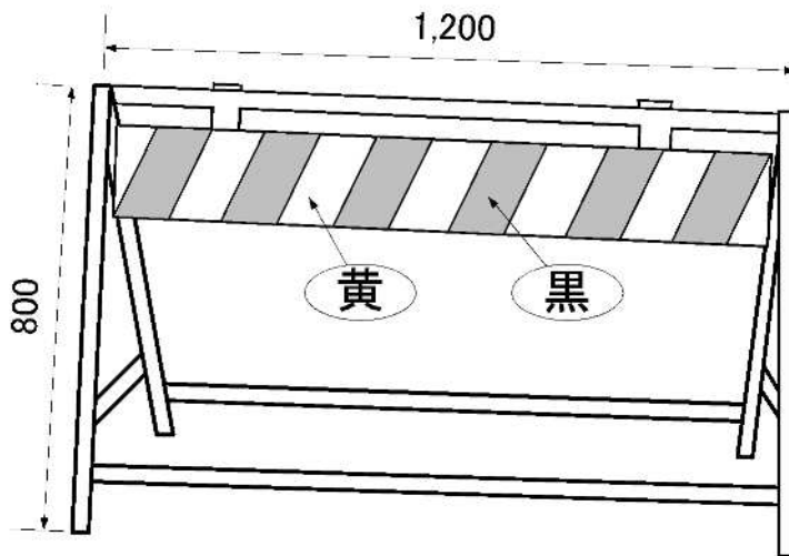
(様式-6) 迂回標示板
