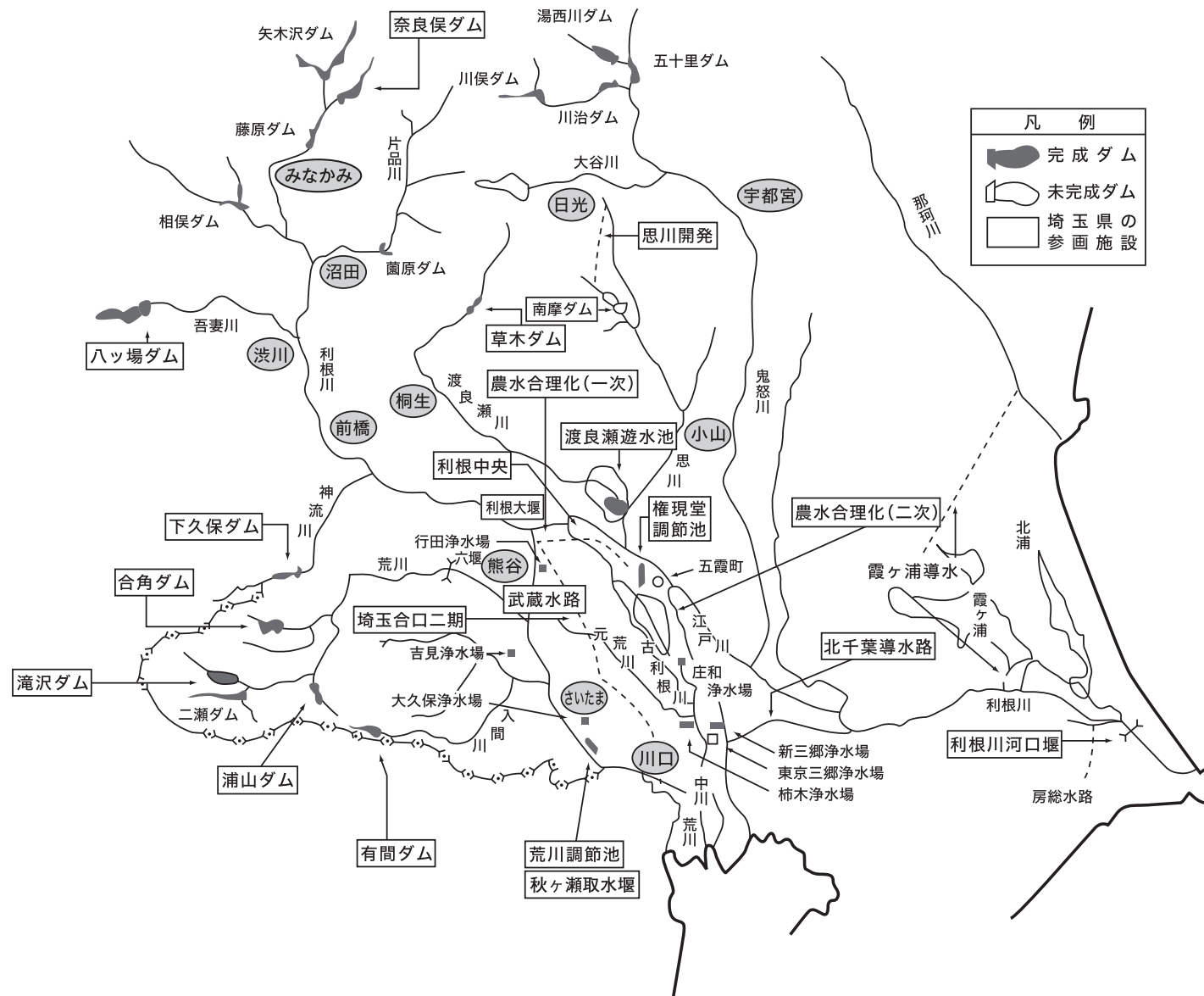
(24) 利根川水系・荒川水系水資源開発施設現況図（令和5年4月1日現在）
