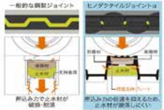
押込み力負荷範囲の比較
