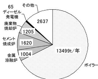
図2 硫黄酸化物排出量(1978年度)
