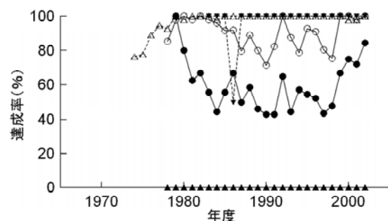
△一般局SO 2 (長期) ▼自排局SO 2 (長期) ○一般局NO 2 ●自排局NO 2 ▲一般局O x
