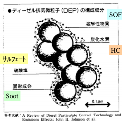
図22 DEPの構造模式図 16)
