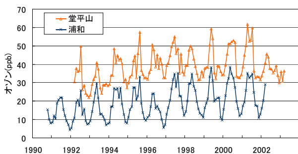
図32 埼玉県内におけるオゾン濃度の推移
