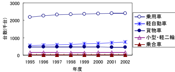
図9 自動車保有台数の推移 7)
