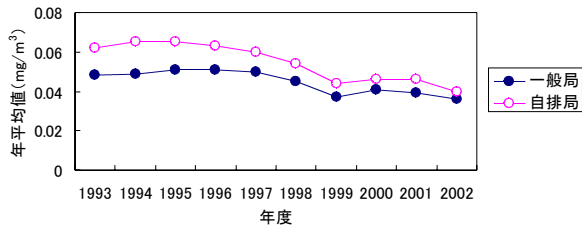
図18 SPM年平均濃度の推移(埼玉県) 17)
