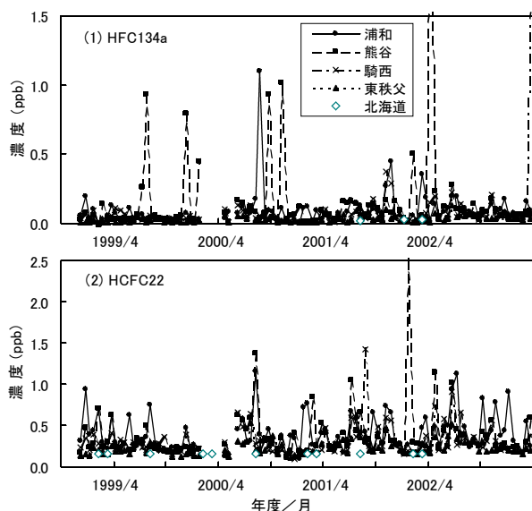
図34 代替フロンの濃度推移
