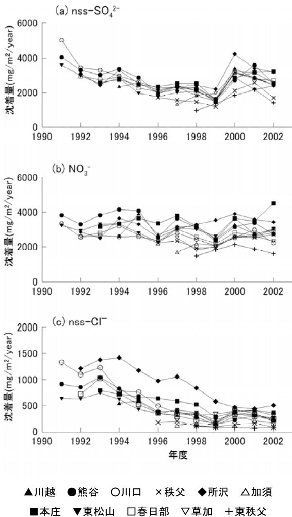
図36 県内各地の湿性沈着量の推移
