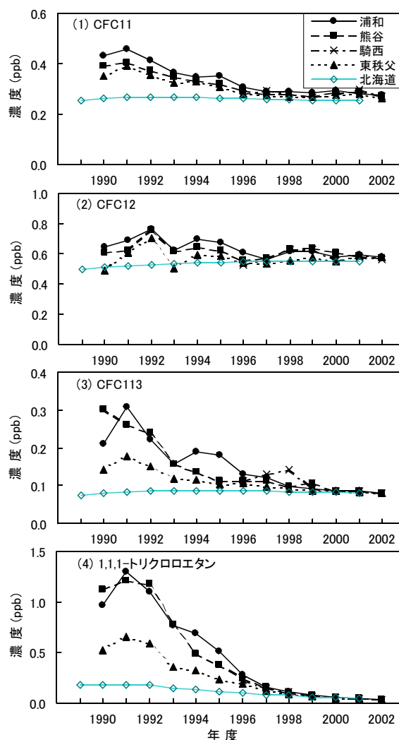
図33 特定フロン類の濃度推移
