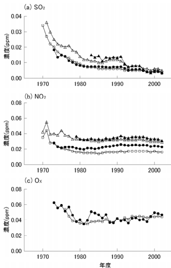
●埼玉県一般局 ○全国一般局 ▲埼玉県自排局 △全国自排局
