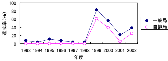
図17 SPM環境基準達成率の推移(埼玉県) 17)
