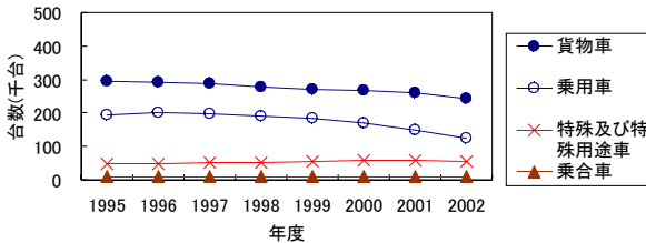
図10 車種別のディーゼル車台数
