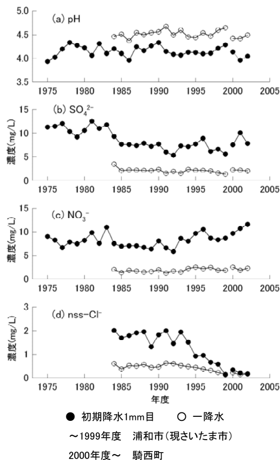
図35 pH及び降水濃度の年度平均値の推移
