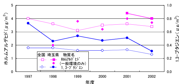
図27 濃度が参考値を上回っていた物質の経年変化
