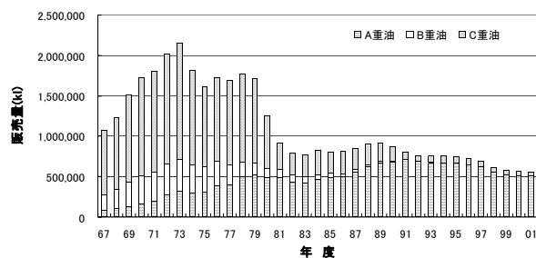
図4 埼玉県における重油の販売量
