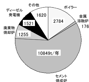
図3 窒素酸化物排出量(1978年度)
