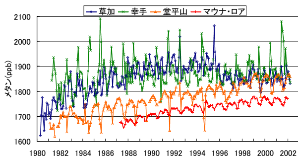
図31 メタン濃度の推移
