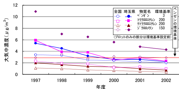
図24 有害大気汚染物質濃度の推移
