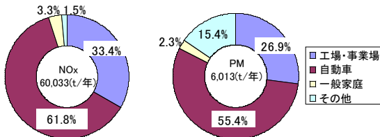
図6 NO x とPMの発生源割合(埼玉県、2000年度) 6)
