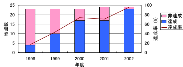
図25 ベンゼン環境基準達成状況の推移(埼玉県)
