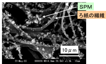
図15 SPMの電子顕微鏡写真
