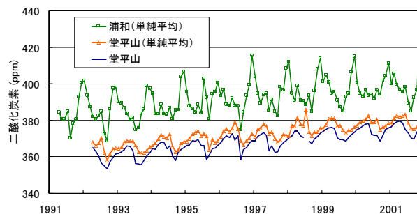
図30 埼玉県内における二酸化炭素濃度の推移
