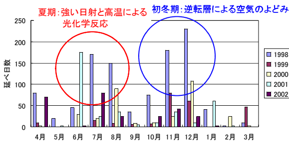
図19 SPM環境基準超過延べ日数(埼玉県) 17)
