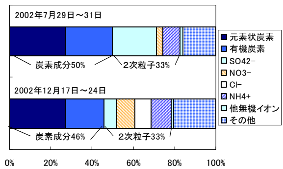
図20 PM 2.5 構成成分割合(騎西町)
