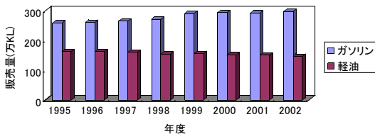
図12 燃料販売量の推移 7)
