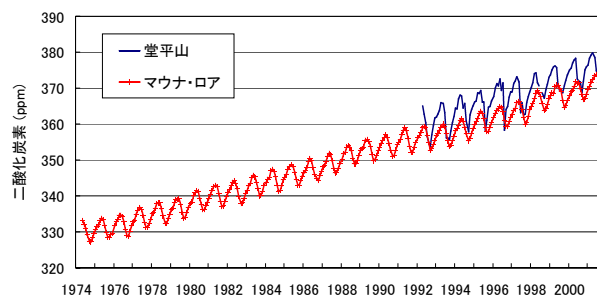
図29 二酸化炭素濃度の推移
