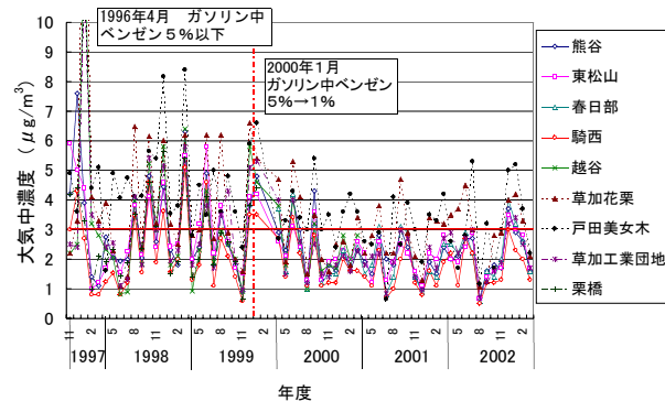
図26 埼玉県測定局のベンゼン濃度
