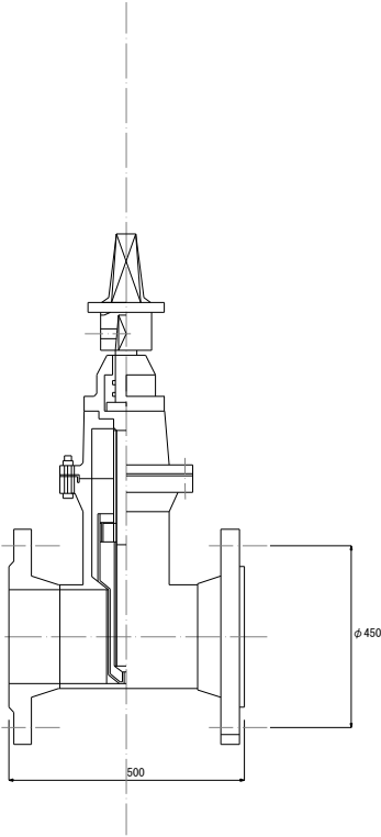
仕切弁標準図 再生水-G2 S=NONE （ソフトシール仕切弁 内ねじ式） 7.5K \phi 450
