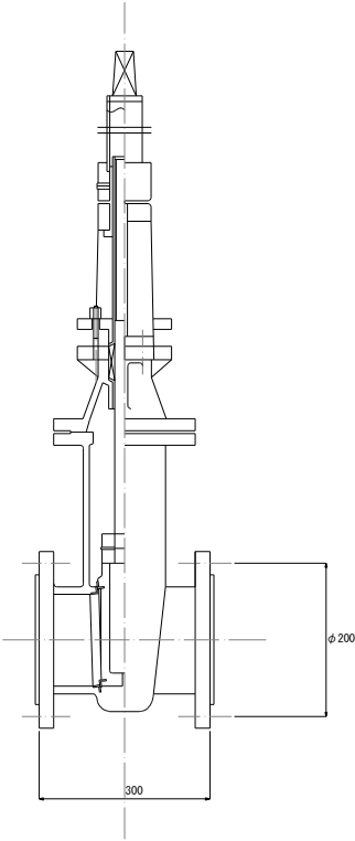
仕切弁標準図 再生水-G1 S=NONE （ソフトシール仕切弁 外ねじ式 7.5K φ200）
