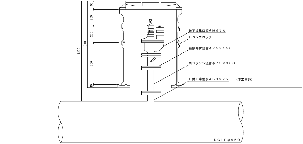
断面図
