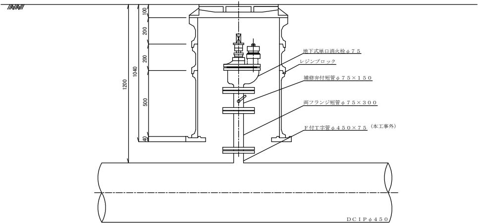
断面図
