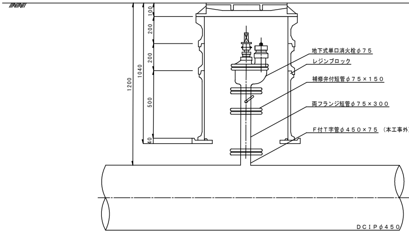
断面図
