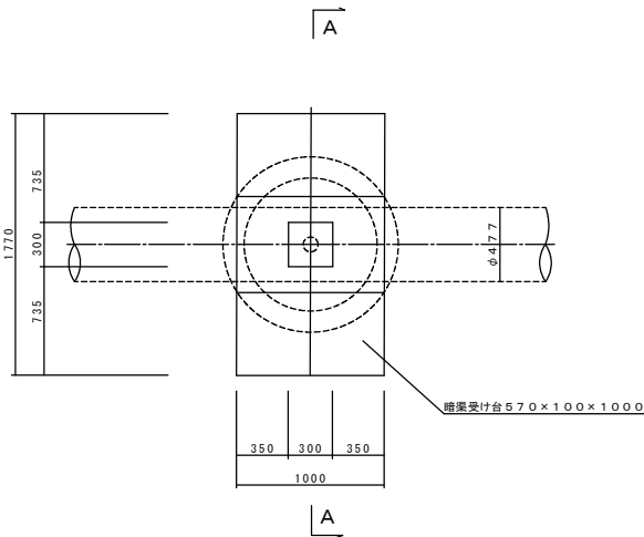
A-A断面図
