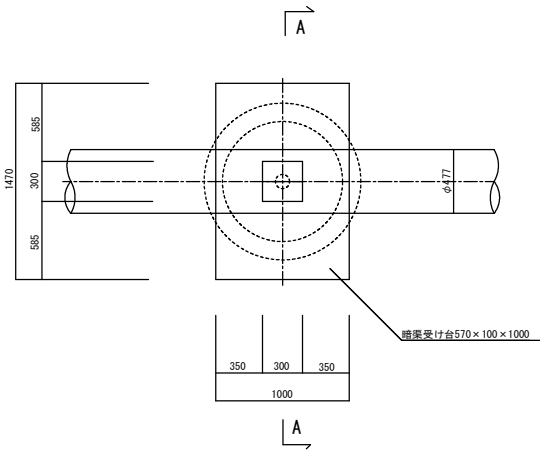
平面図
