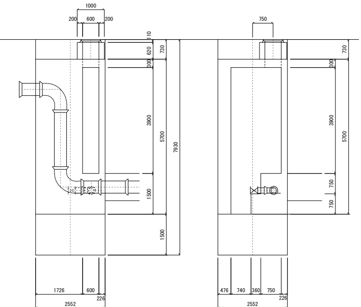
①-①断面図
