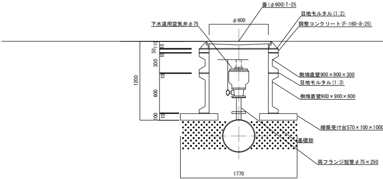
A-A断面図
