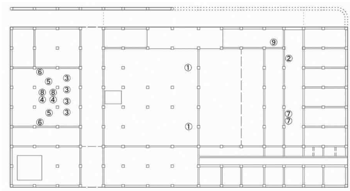
図 9.3-9(1) 振動源となる主要な設備機器の配置 (新焼却処理施設 1 階)
