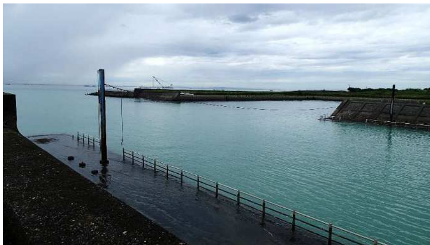
図 1-3 青潮状態の境川河口(写真左奥が東京湾)
