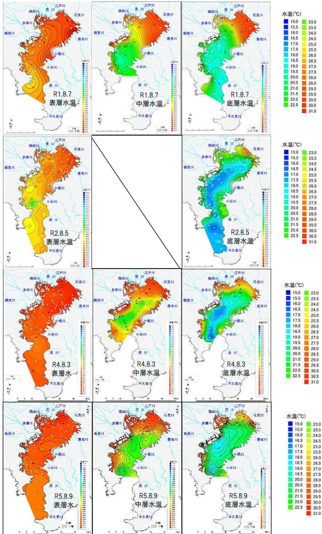
図 6-1c 令和元年から令和 5 年(令和 3 年を除く) 8 月における東京湾の水温の状況
