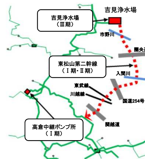
吉見浄水場拡張関連整備事業 全体図
