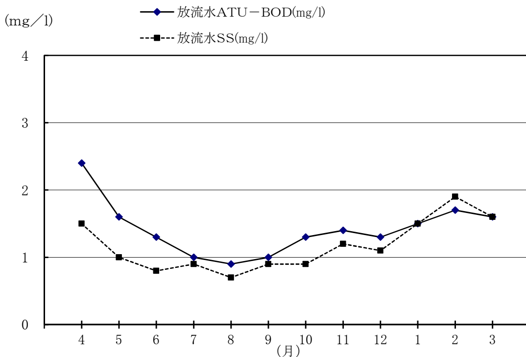
図6-8 令和3年度 放流水 BOD・SS
