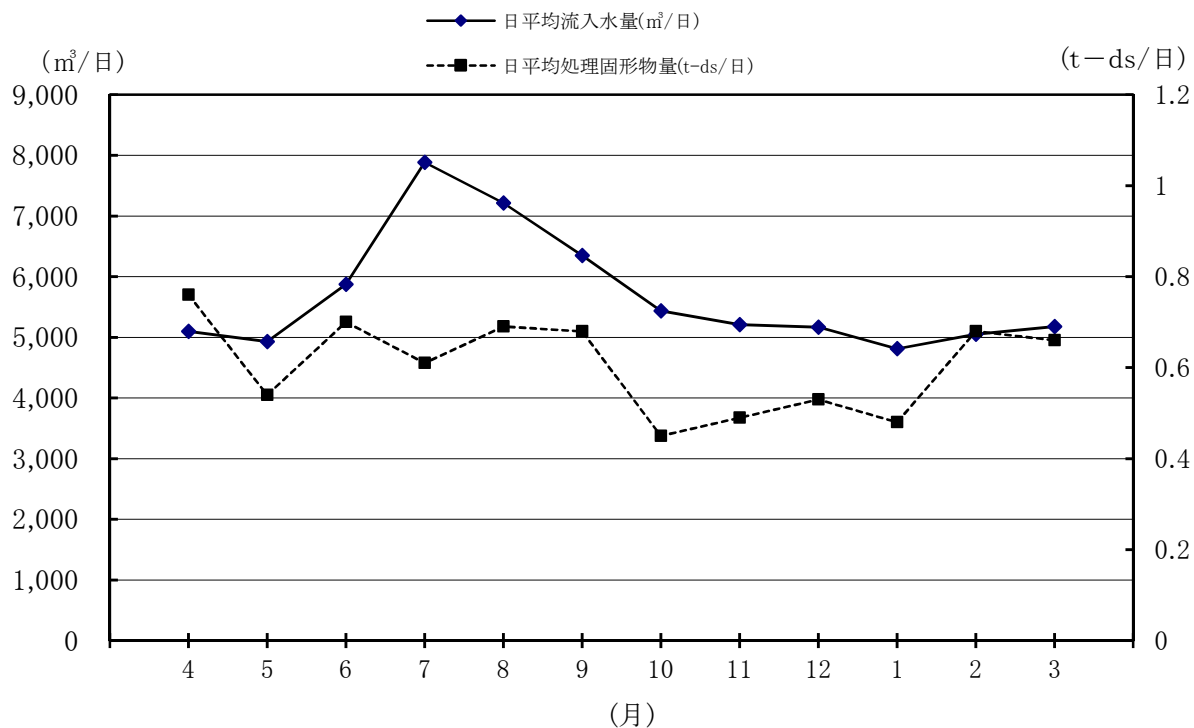
図6-7 令和3年度 流入水量・処理固形物量
