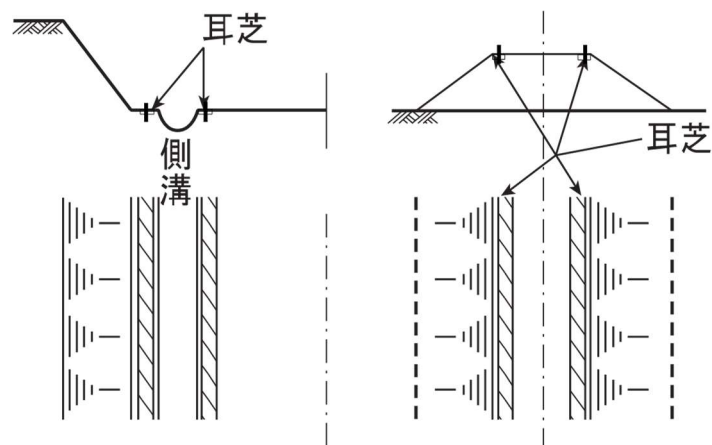
図3-2-6 耳芝
