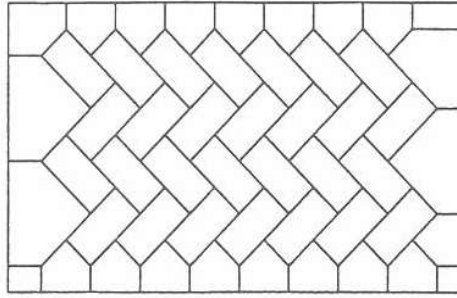
図3-2-4 谷積
