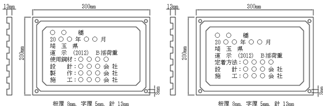
図3-2-2 銘板の寸法及び記載事項
