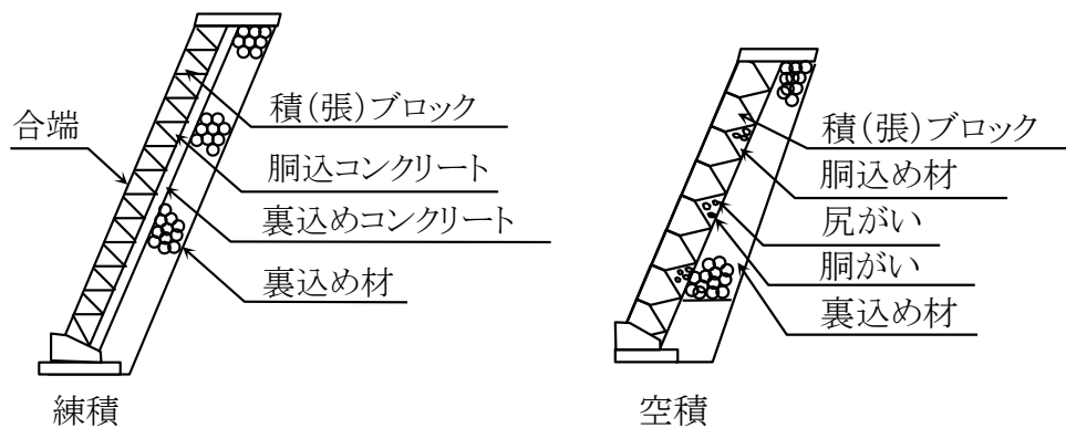
図3-2-5 コンクリートブロック工（標準図）
