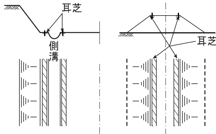
図3-2-6 耳芝
