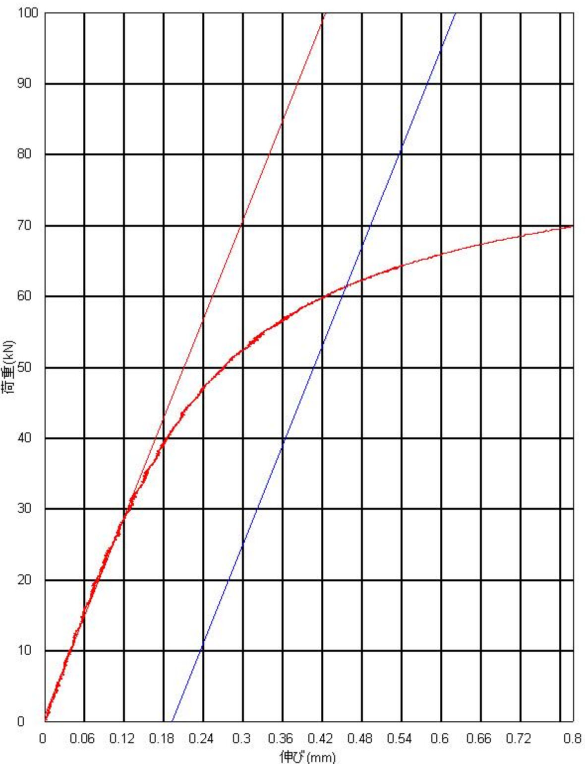
0.2%耐力線図
