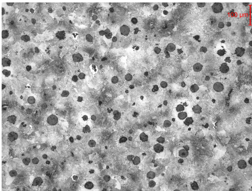
サンプル名 : 球状黒鉛鑄鉄 エッチング液 : 5%ナイトル 撮影倍率 : 100倍
