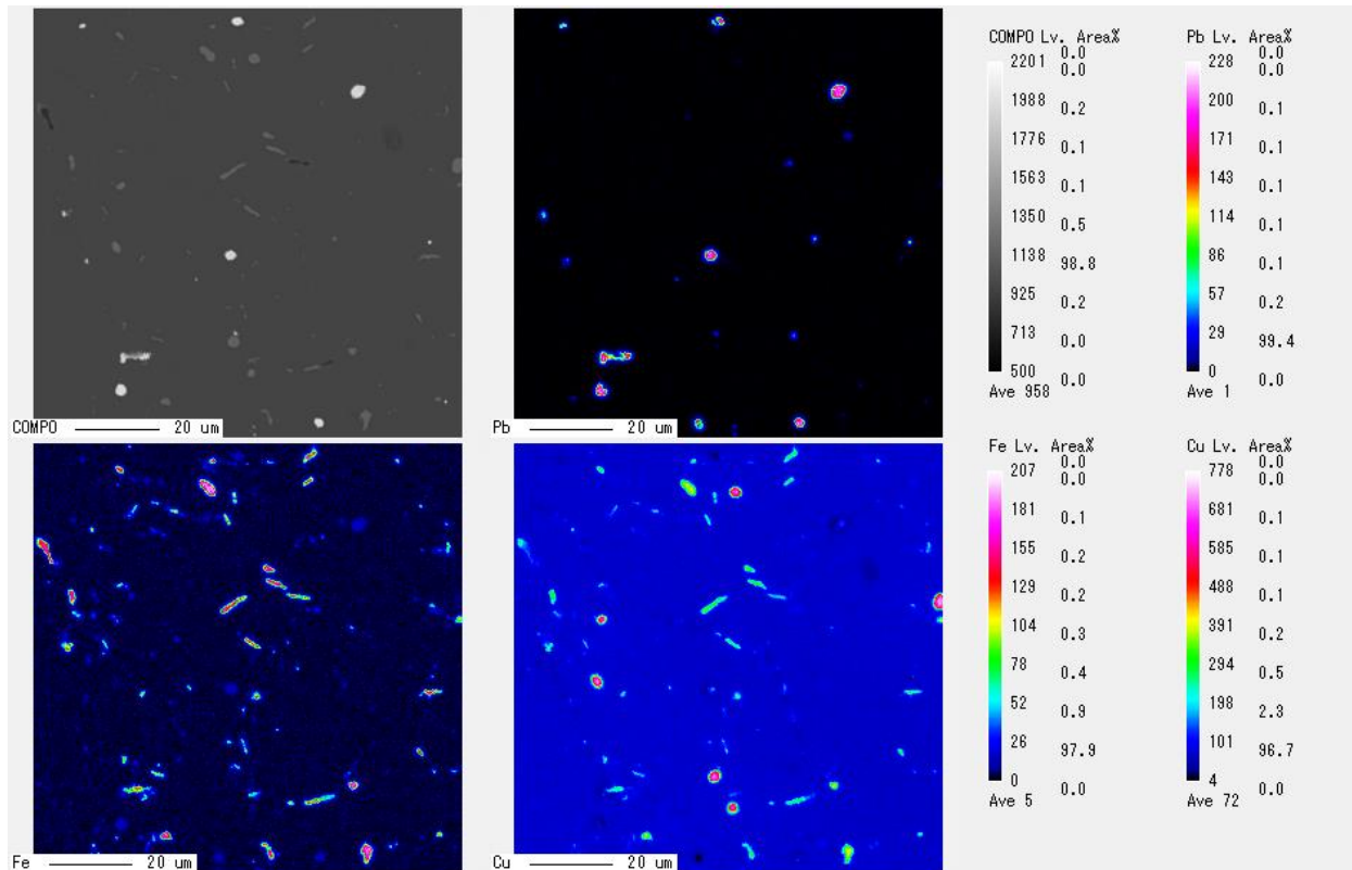
図：X線マイクロアナライザのカラーマップ(成績書別紙)
