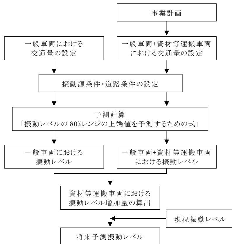
図 9.3-3 工事中の資材運搬等の車両の走行に伴う振動の予測手順
