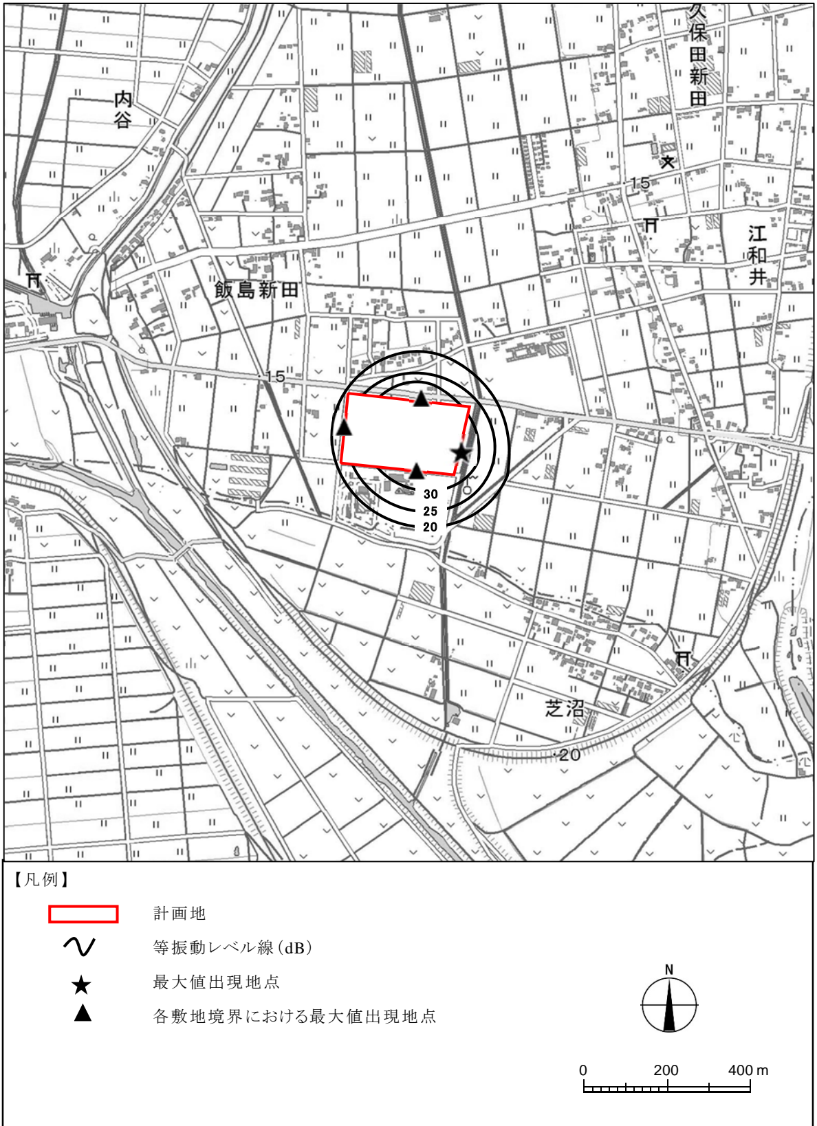
図 9.3-7 寄与振動レベル分布図 (L 10 : 昼間)
