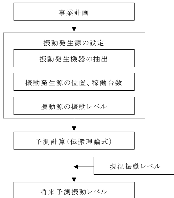
図 9.3-4 供用後の施設の稼働に伴う振動の予測手順
