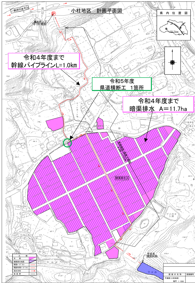
小柱地区 計画平面図
