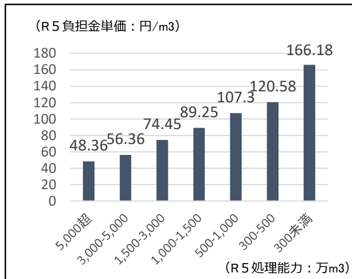
全国流域下水道の処理規模別負担金単価(処理区単位)
