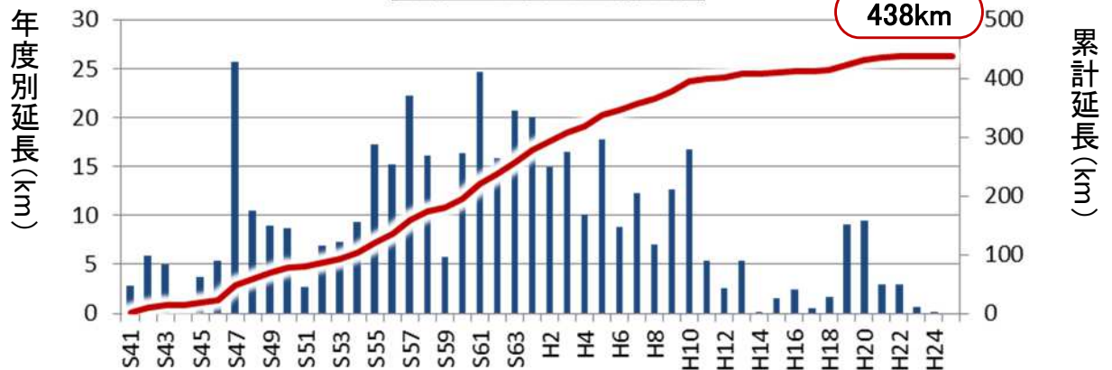
管渠の年度別整備延長
